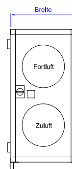
rechte Seite
