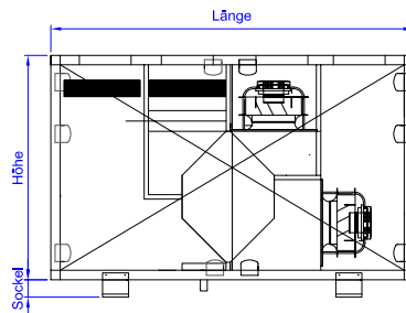
Ansicht Revisionsseite
