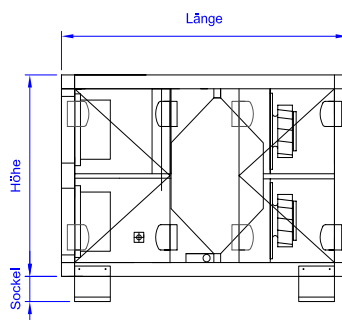
Ansicht Revisionsseite
