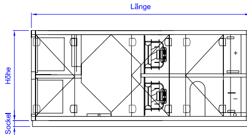
Ansicht Revisionsseite
